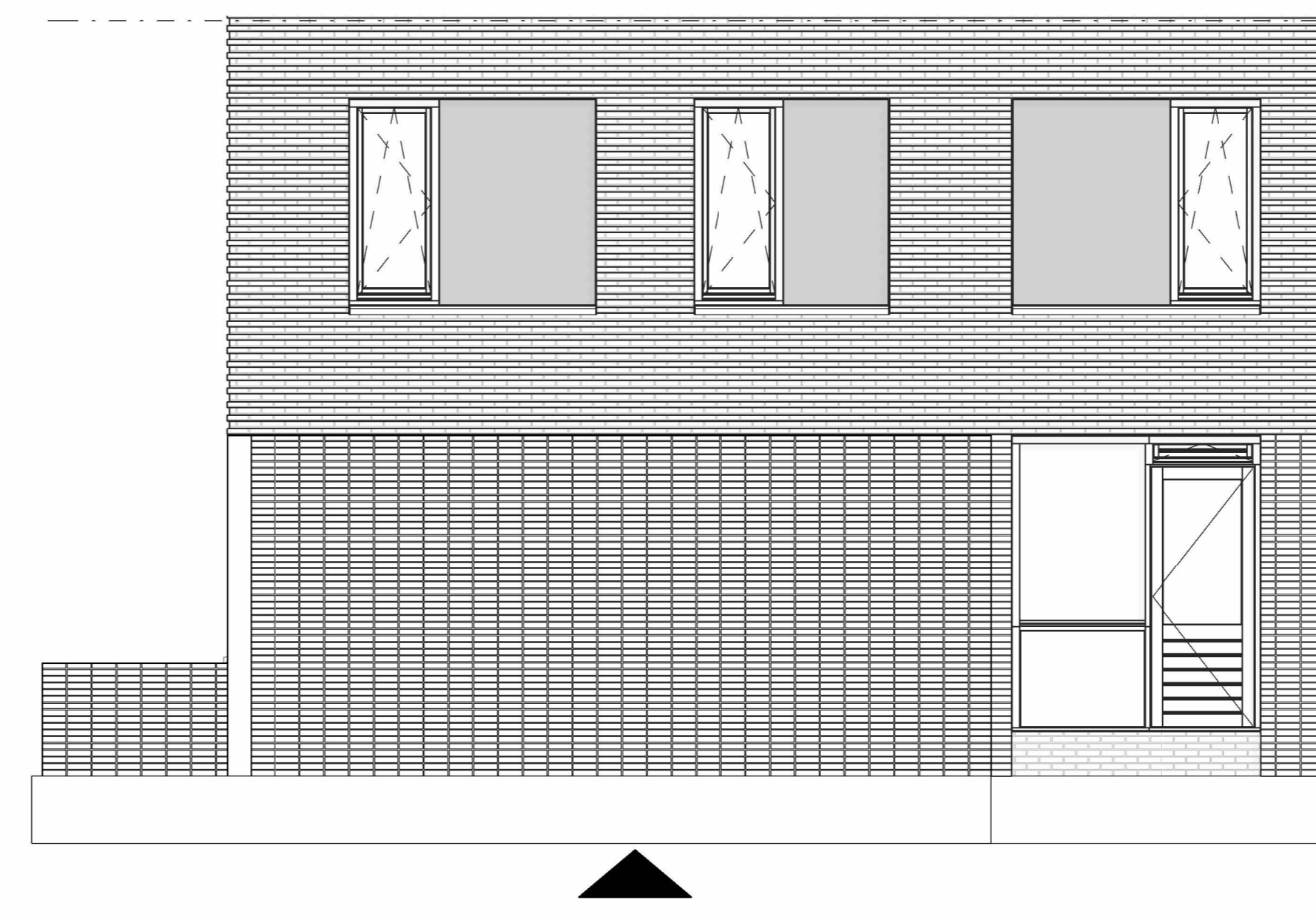
achtergevel / muur
