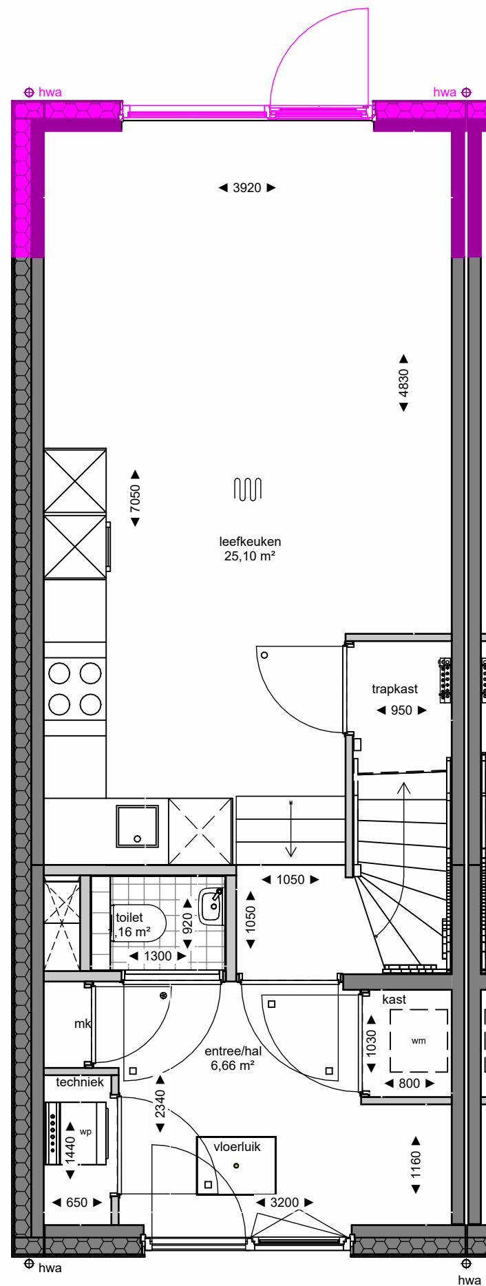
Begane grond
