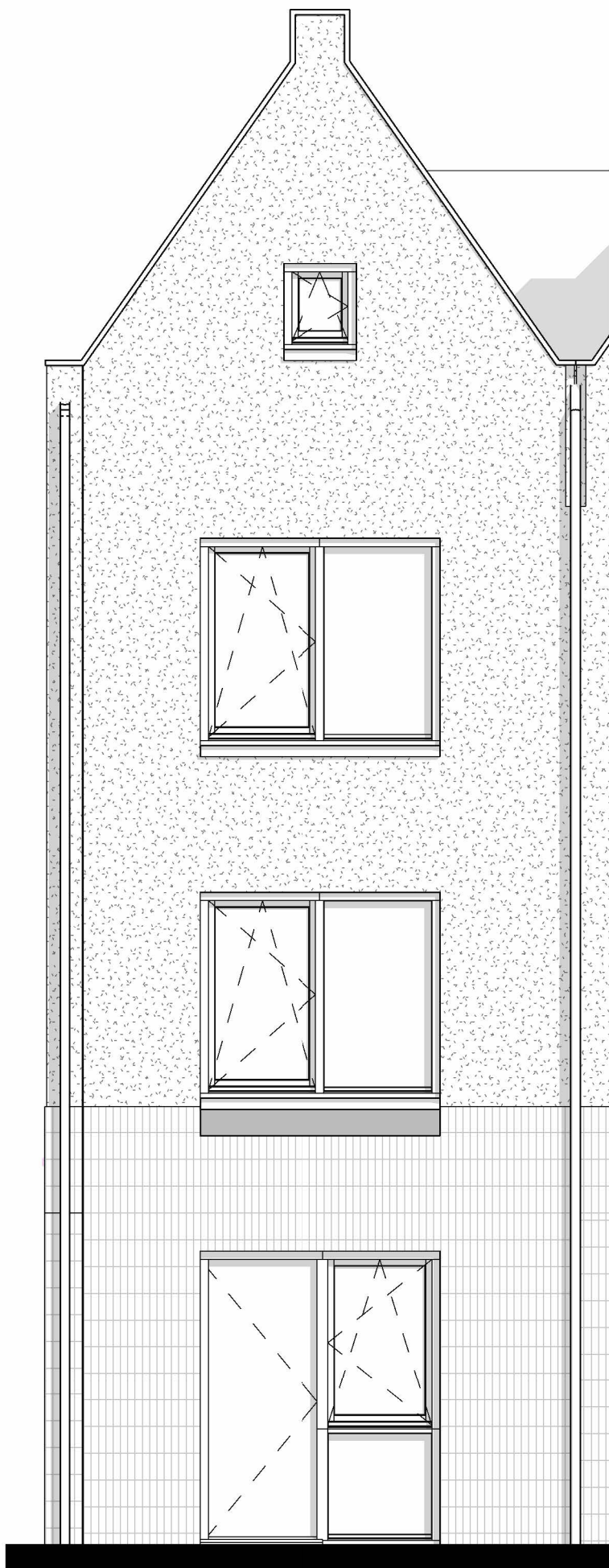
voorgevel
