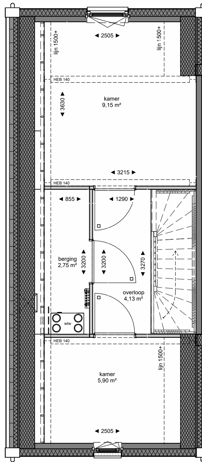
3e verdieping
