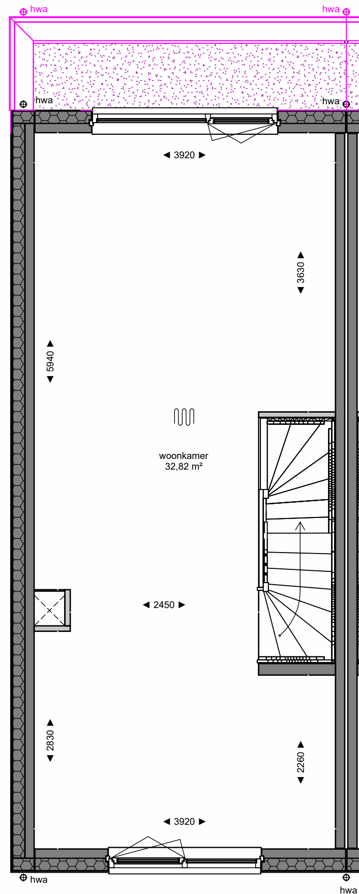
1e verdieping
