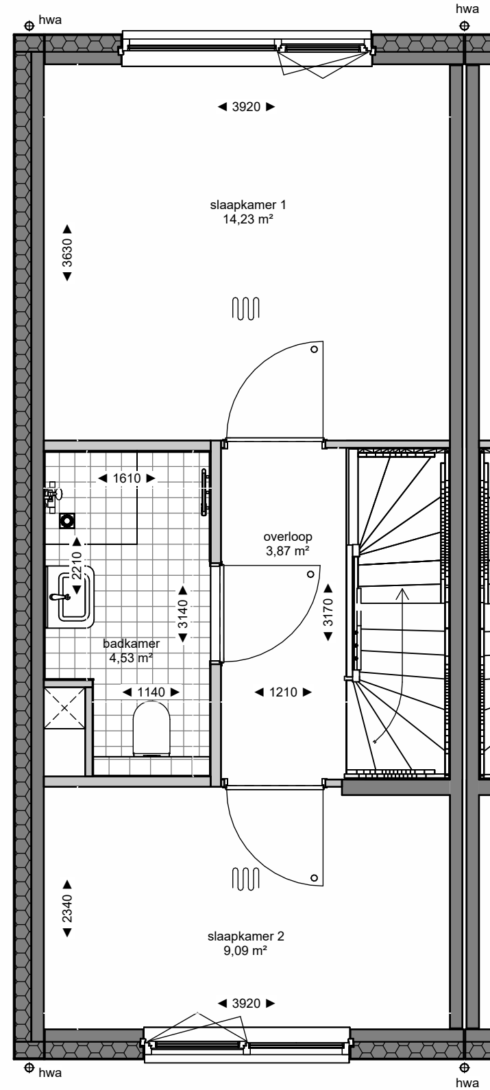
2e verdieping
