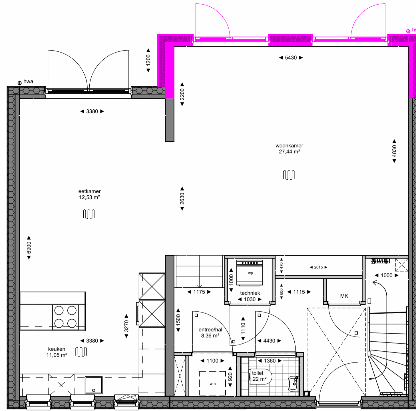
Begane grond
