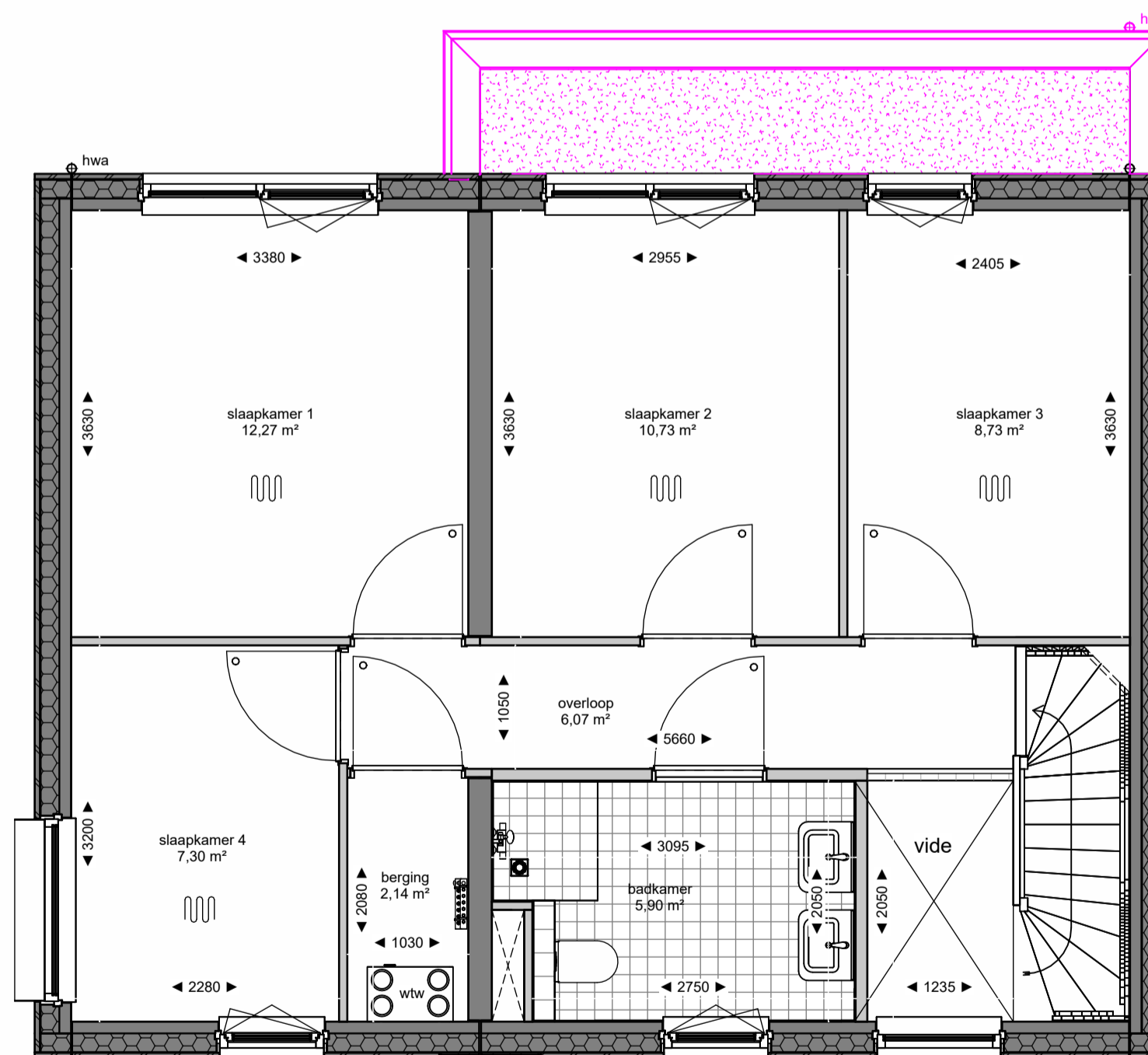
1e verdieping
