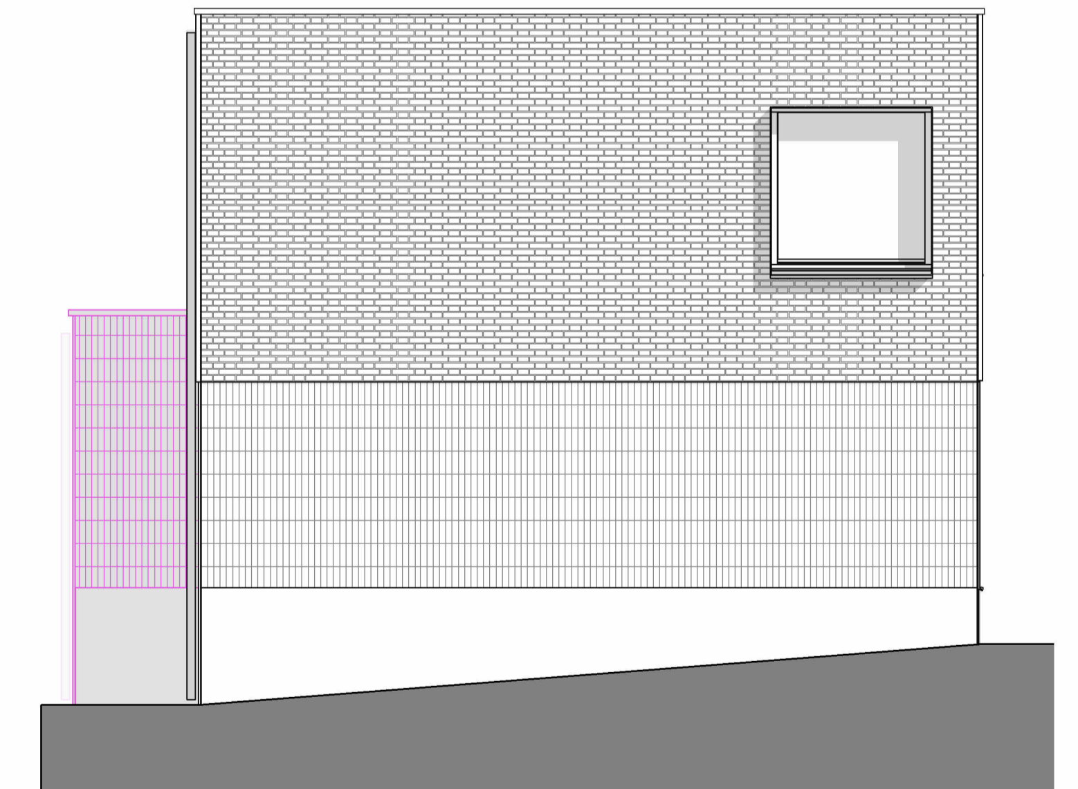
linker zijgevel
