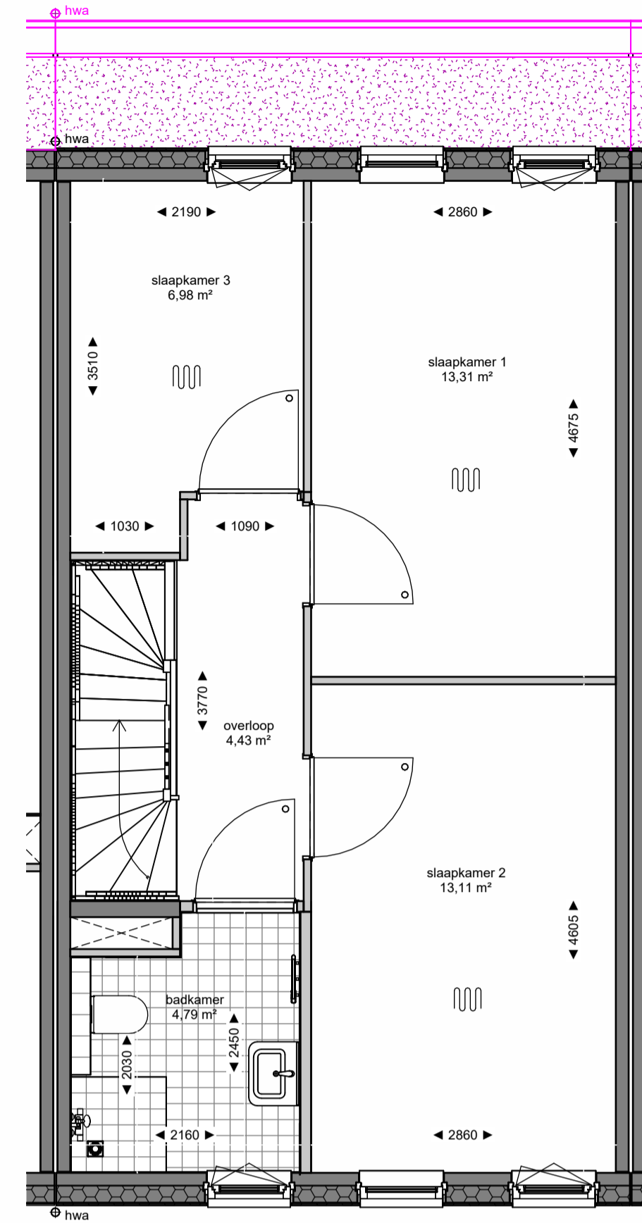
1e verdieping
