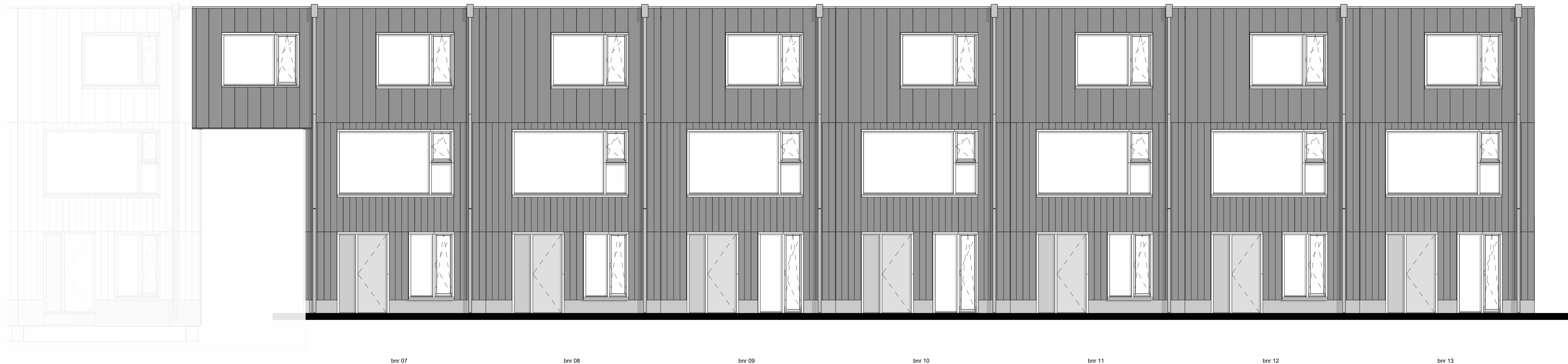
voorgevel
